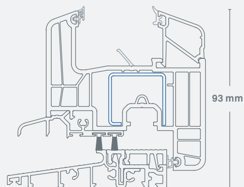
Barrier-free balcony door threshold Fig.: 1:2
